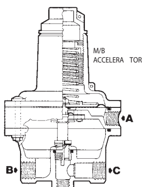
A = Выходное давление - Downstream pressure B = Давление от пилота - Motorization C = Выход газа - Exhaust
